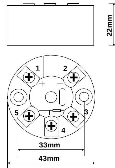
Rys.1.Nagłowicowy Mikroprocesorowy Przetwornik Temperatury GMPT-01 - wymiary.
