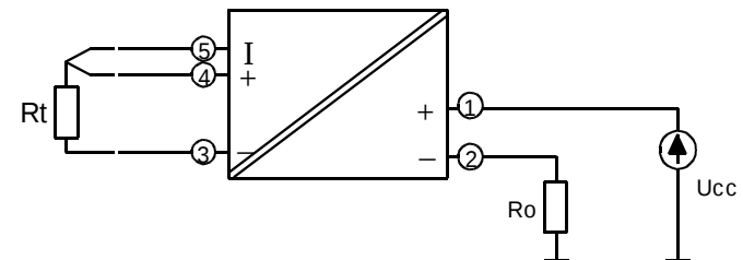
Rys.2.Schemat podłączenia przetwornika GMPT-01.
