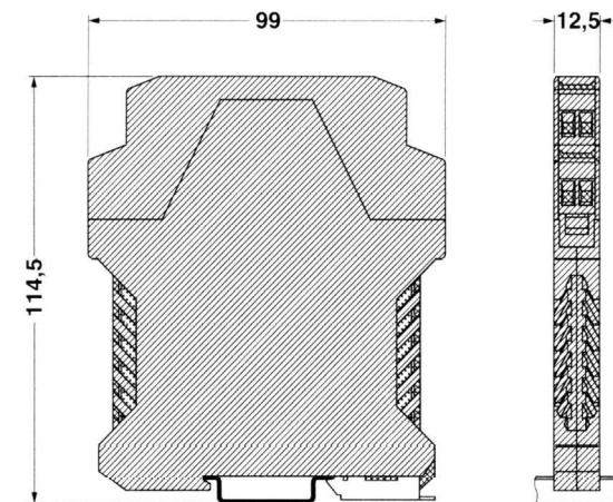
Rys.1.Listwowy Powielacz Sygnałów Analogowych LPSA-11ME - wymiary.
