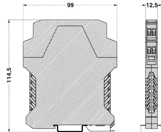
Rys.1.Listwowy Uniwersalny Przetwornik Sygnałowy LUPS-11ME - wymiary.
